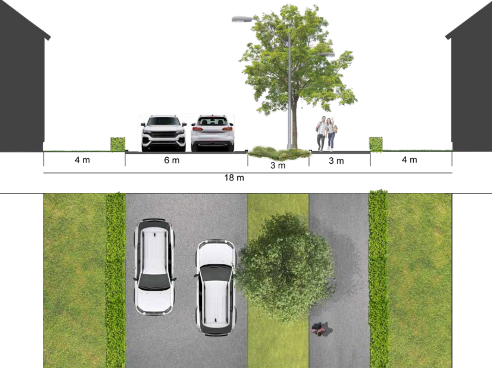
Exempel på gatusektion över Huvudgatan i Kvarnåker.
