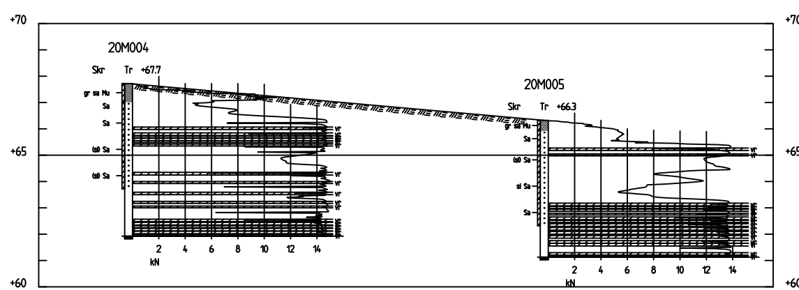
SEK션 B-B H 1: 100 L 1: 400
