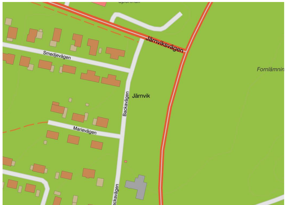
▲ Utdrag ur SGU:s jordartskarta, Isälvsediment
