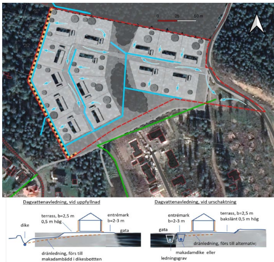
Figur 19. Figur som redovisar ett förslag på uppsamling av dagvatten med små diken/ledningar visas schematiskt med ljusblå linjer utifrån erhållen situationsplan. Grön linje visar ungefärligt läge för befintlig dagvattenledning och dike för den redan färdigställda dagvattenavledningen.
